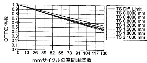
FIG. 6C
